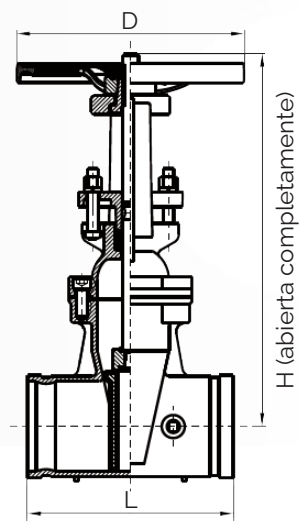
FIGURA 1: Dimensiones
